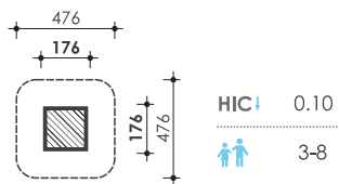
Sklepik z tablicą do rysowania PD/PM 2004
