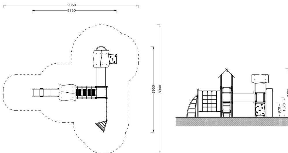
RZUT I ELEWACJA
